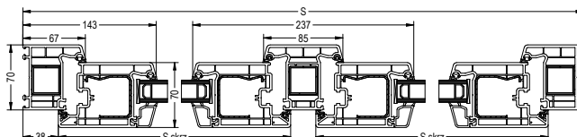
Sezione orizzontale anta larga
